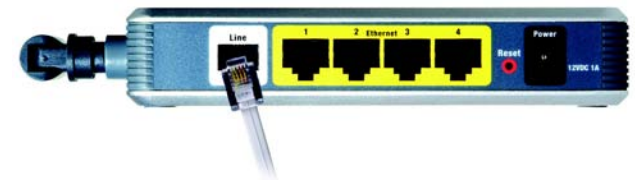
Figure 4-4 : Connexion de la ligne ADSL
